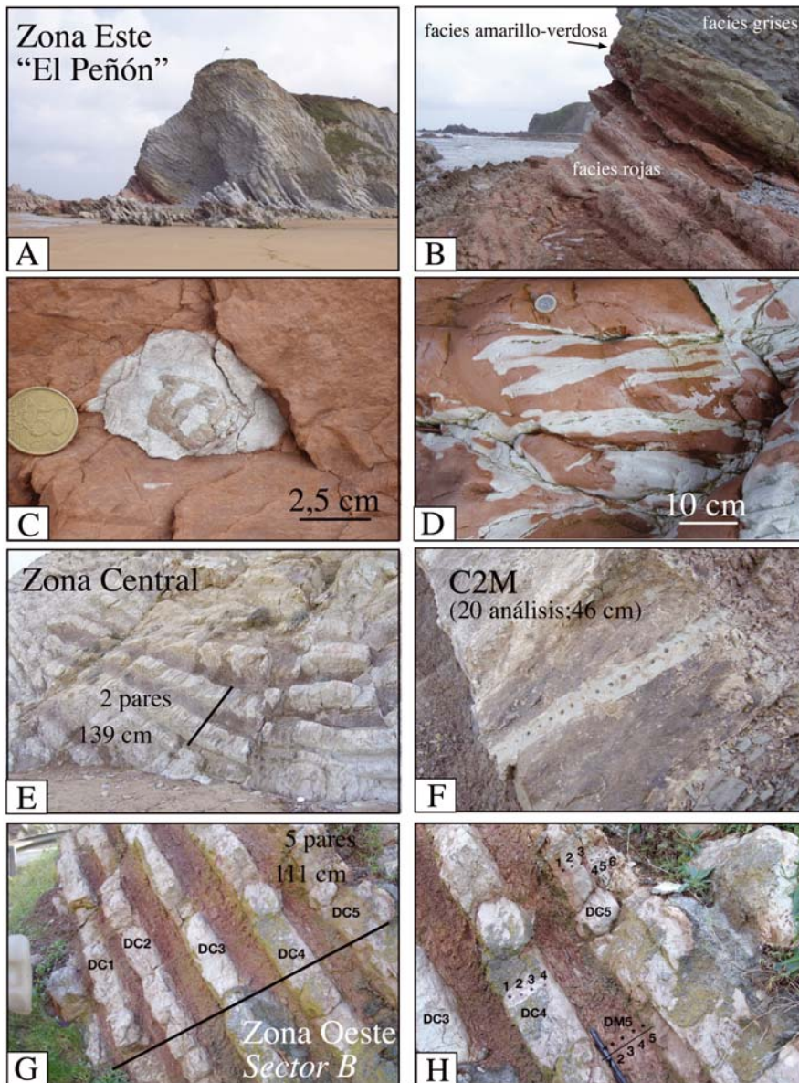
Fig. 1.- Sección de Sopolana con las zonas estudiadas. Explicaciones en el texto.
